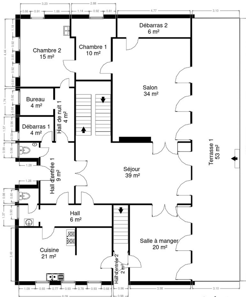
Rez-de-chaussée
